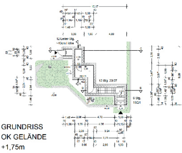
GRUNDRISS OK GELÄNDE +1,75m
