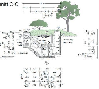
Schnitt C-C
