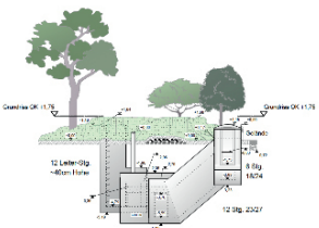
Ansicht Süd-Ost
